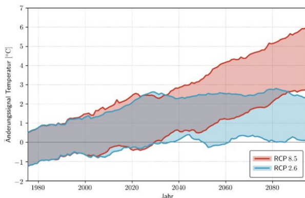
Die zu erwartenden Temperaturänderungen in Deutschland bis zum Ende dieses Jahrhunderts. RCP8.5: „Weiter wie bisher-Szenario“, RCP2.6: „Klimaschutz-Szenario“ (s. http://reklies.hlnug.de ).
